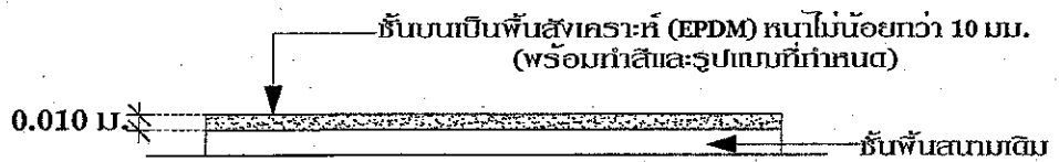
รูปตัดพื้นสนาม A-A
